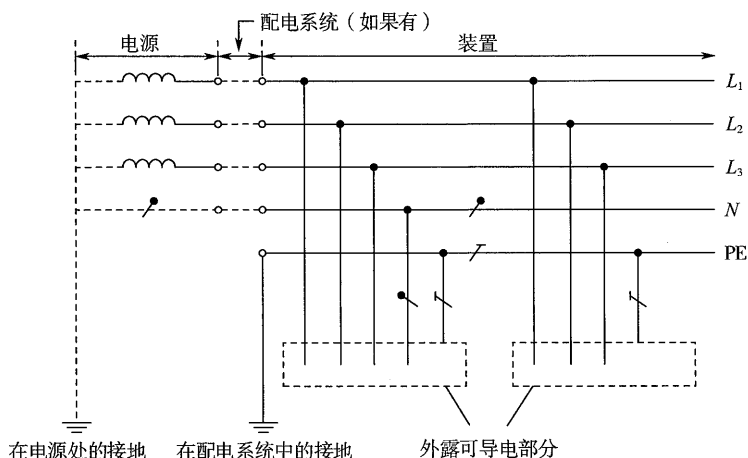
图 3 全部装置都采用分开的中性导体(N)和保护导体(PE)的 TT 系统
