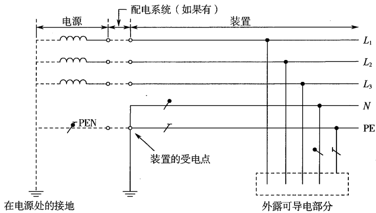
图 2 在装置的受电点将保护接地中性导体(PEN)分离成保护导体(PE)和中性导体(N)的三相四线制的 TN-C-S 系统
