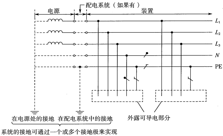
图 1 全系统将中性导体(N)与保护导体(PE)分开的 TN-S 系统
